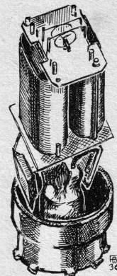
Abb. 3. Die nämliche Röhre enthält zwei getrennte Dreipol-Systeme.
