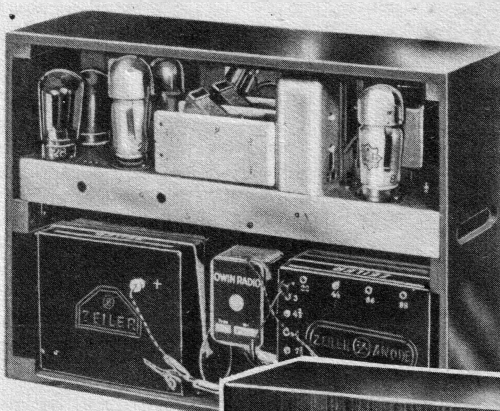
Links: Im Gehäuse oben das Gerät selbst, unten Lautsprecher, Heiz- und Anodenbatterie. Ein Blick in einen Kofferempfänger von rückwärts.
