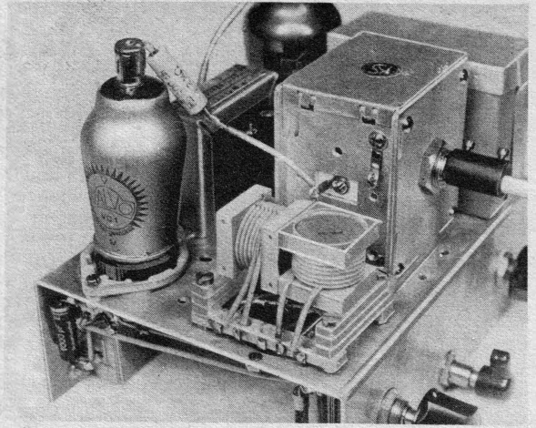
Die Spulen sind besonders deutlich zu sehen. Die Gitterkombination ist unmittelbar am Gitterclip der Audionröhre angebracht. Die Kondensatorachse rechts ist durch eine Isolierkupplung tromlos gemacht.
