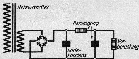
Abb. 2. Die Vorbelaftung kann auch durch den in Abb. 1 ange-deuteten Spannungsteiler dargestellt werden.
