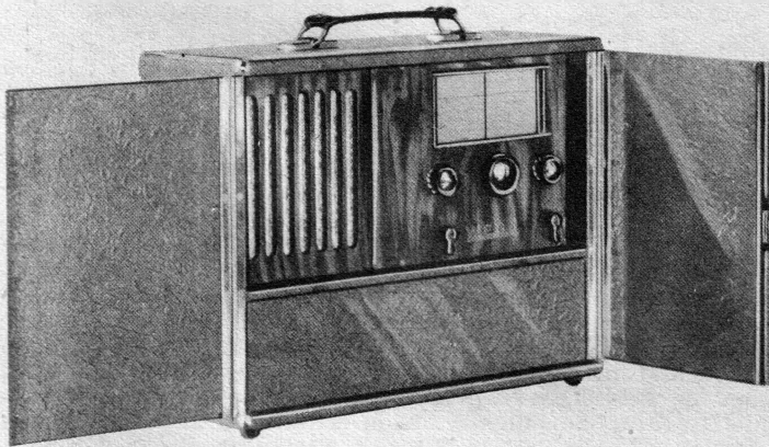
Ein Kofferempfänger mit Türen. Links der Lautsprecher, rechts das Gerät. Werkphoto Wega.
