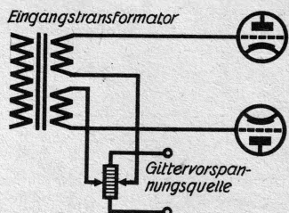
Abb. 1. So läßt sich jede Ungleichheit der Röhren reiflos ausgleichen.
